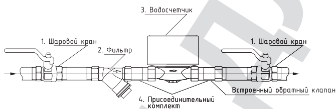
Рекомендуемая схема водомерного узла:
